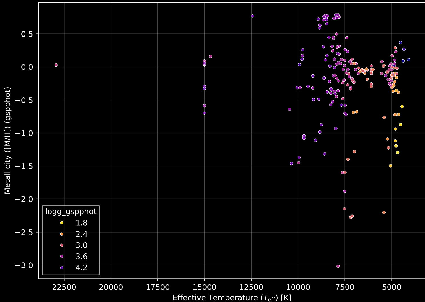
APOGEE DR17 Field: [270-04] Stellar Population Parameters (n= 221)
